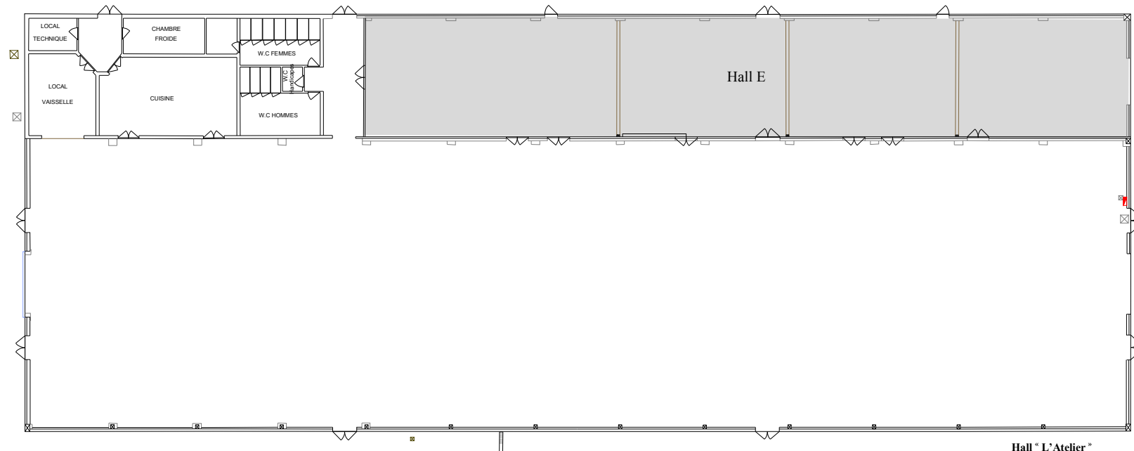
Hall " L'Atelier " Echelle 1/250 Côtés intérieures : 77m50 / 19m60
