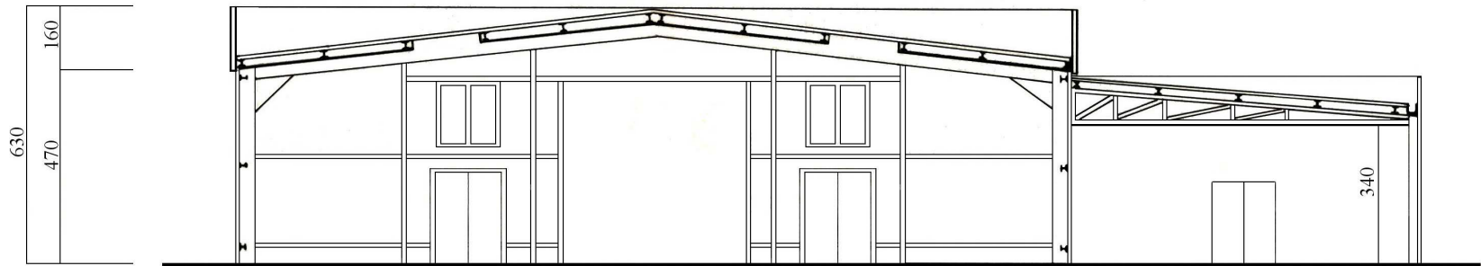
PLAN DE COUPE HALL A
